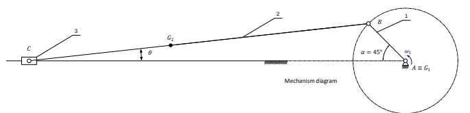
Hình 6: Sơ đồ nguyên lý của cơ cấu tay quay con trượt tại vị trí 45°
